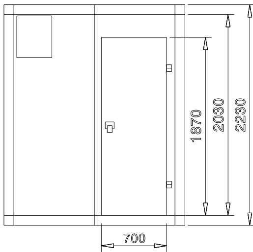
Zij aanzicht
