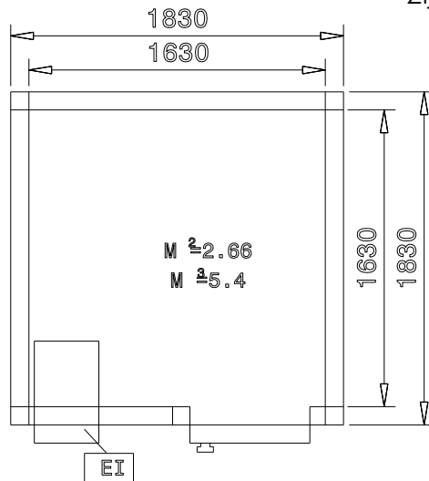
Boven aanzicht
